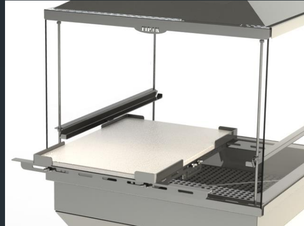
Beispiel: Lavastein für Pizza & Flammkuchen (Sonderzubehör*)
